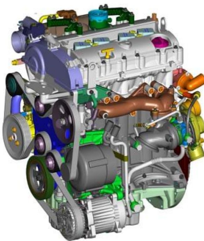
موتور EF7
